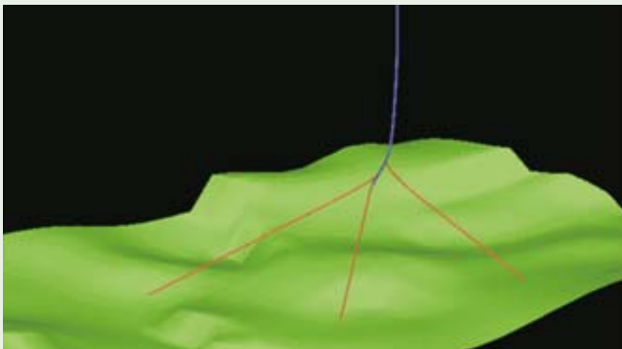
На схеме многоствольная конструкция скважины №5887.
